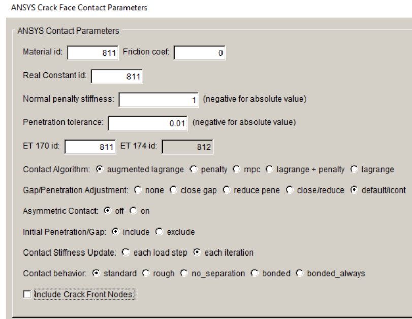
Figure 13.9 ANSYS CFC parameters dialog.
